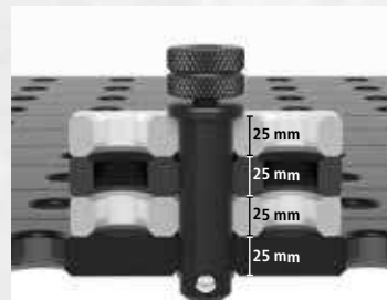
Varžtas keturgubas
